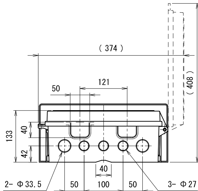
底面図 (1/6)
